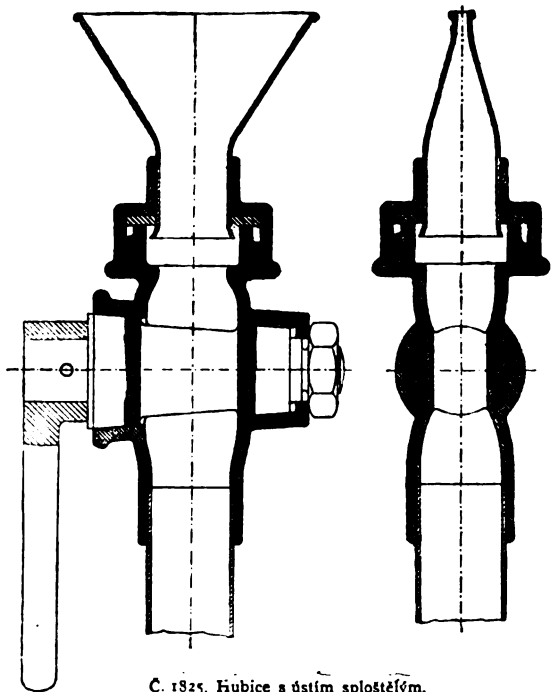
C. 1825. Hubice s ústím sploštělým.
